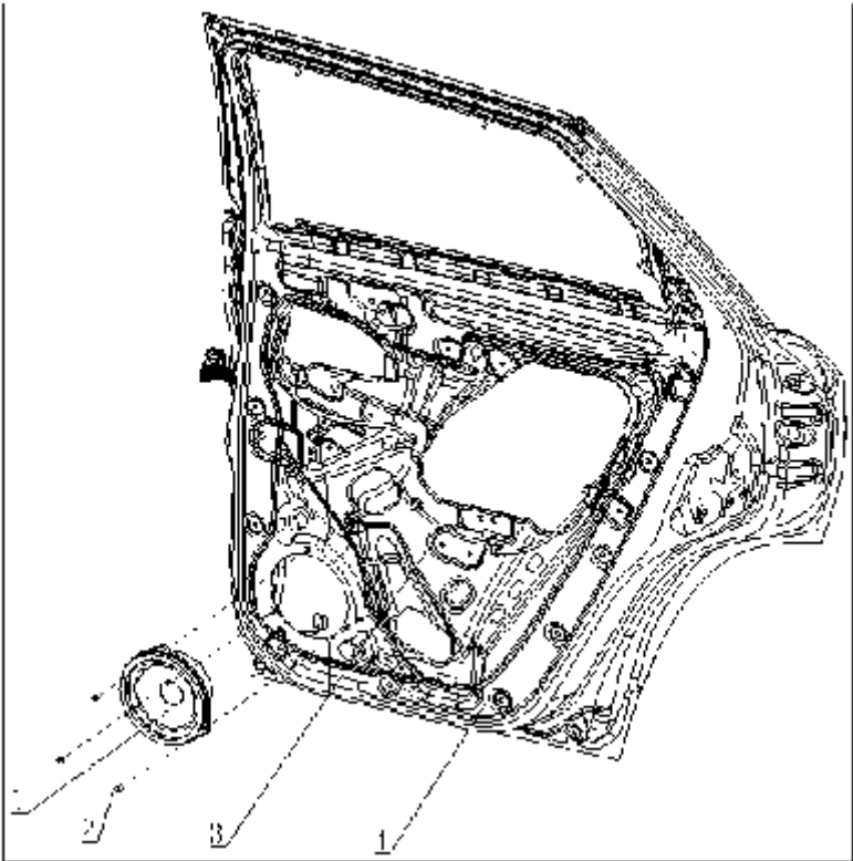
后门扬声器部件视图
